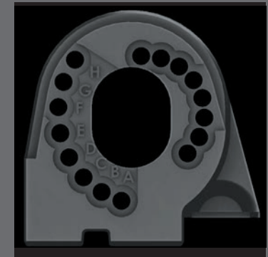
Posiciones de los tornillos
